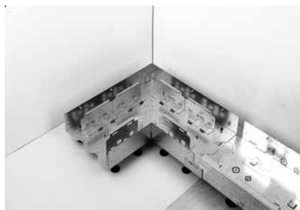
3. Les socles de la goulotte sont assemblés au moyen de jonctions et les extrémités de la goulotte sont couvertes avec des plaques de fermeture. Il est impératif que la chape ne rentre pas dans la goulotte. Les vis fournies sont utilisées pour établir une liaison électrique entre la jonction et les socles.
