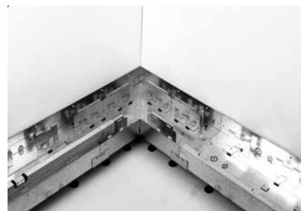
4. Ajustage de la hauteur de la goulotte qui définit la hauteur de la chape. Il est recommandé que le montageur se mette en contact avec l'électricien qui réalise cette dernière. Recommandation minimale : 4 vis de nivellement par mètre.
